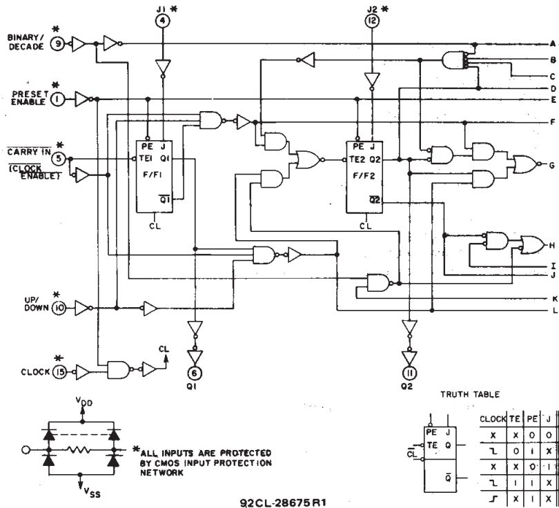
Fig. 9 - Logic diagram.
